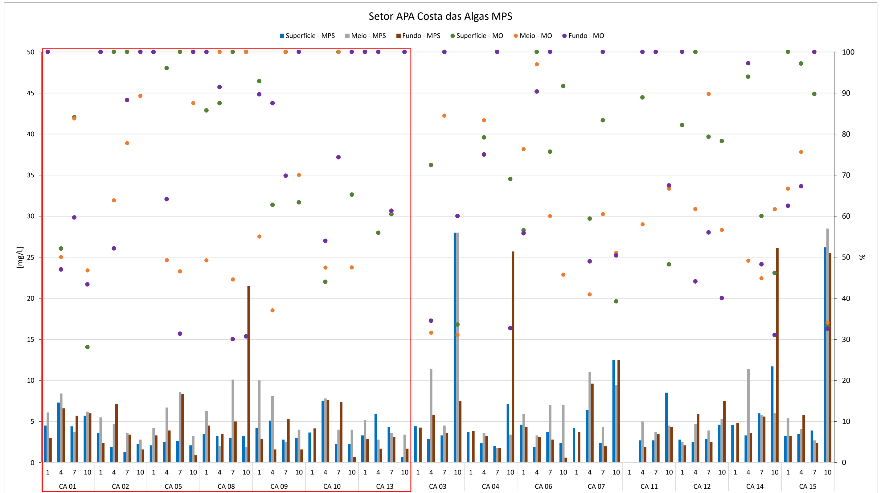
Figura 58: MPS e os respectivos teores de MO da camada superficial, meio e fundo da coluna d'água do Setor APA Costa das Algas. As estações rasas se encontram dentro do quadrado vermelho.
