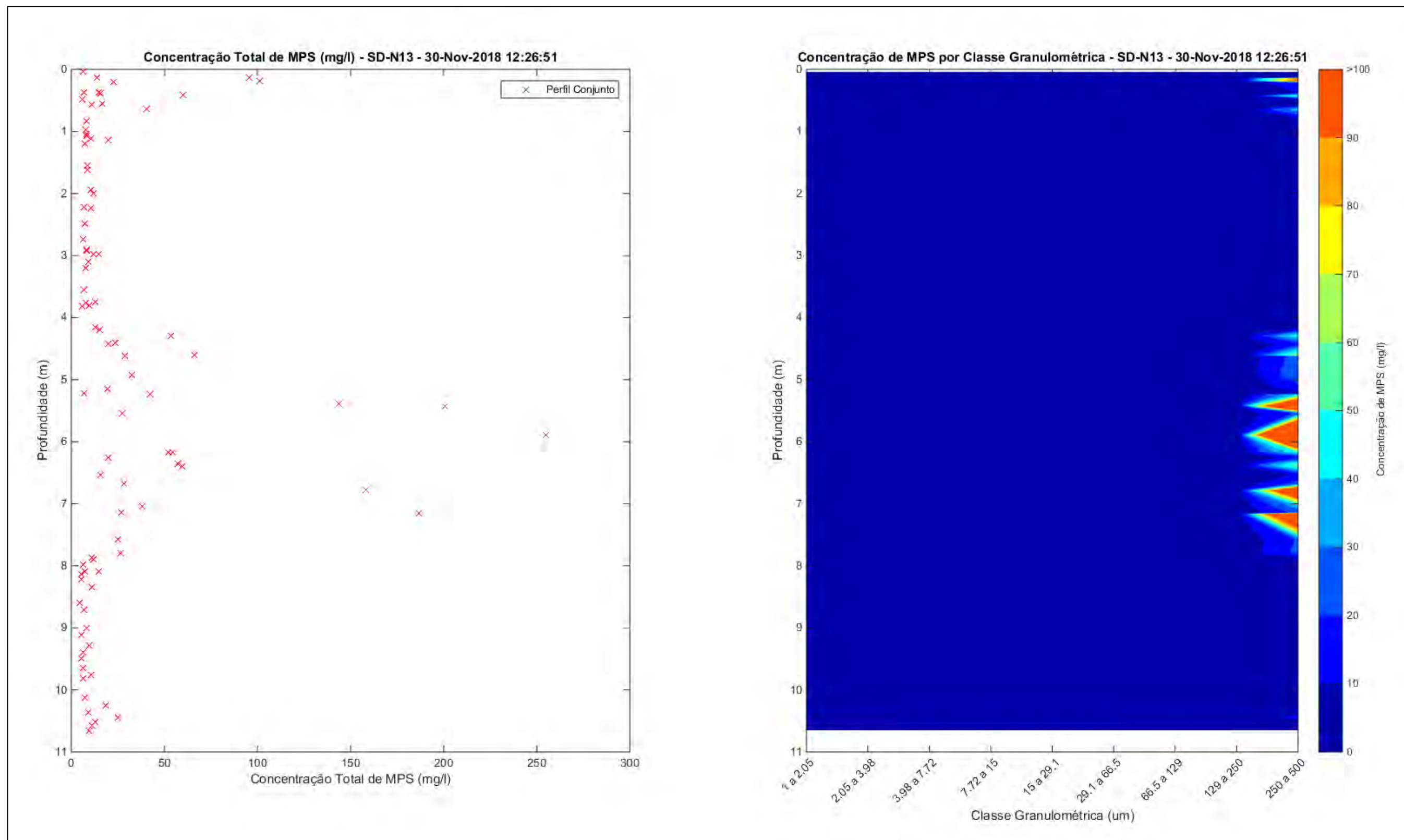
Apêndice 2: Perfis realizados pelo LISST na Campanha 2.
