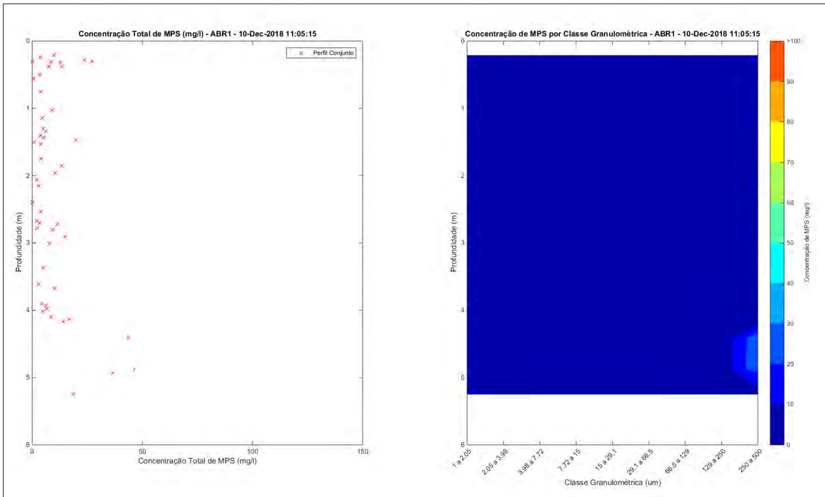
Apêndice 1: Perfisagens realizadas pelo LISST na Campanha 1.
