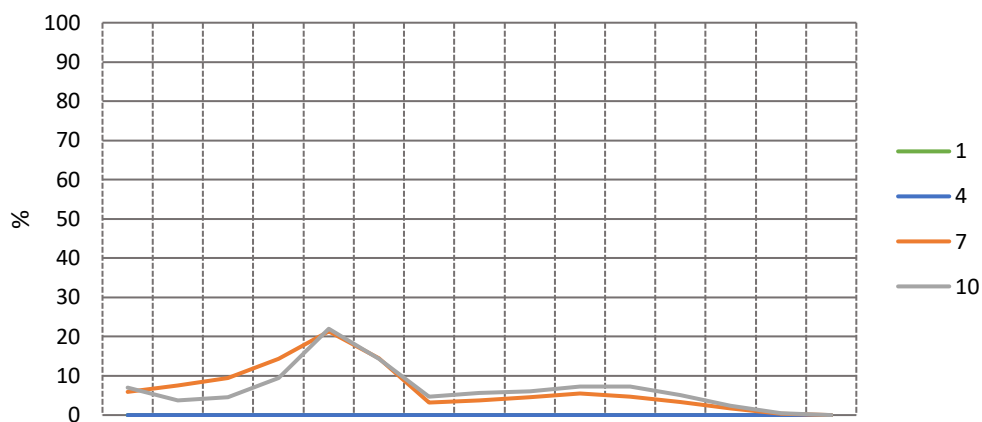
Granulometria CA 10
