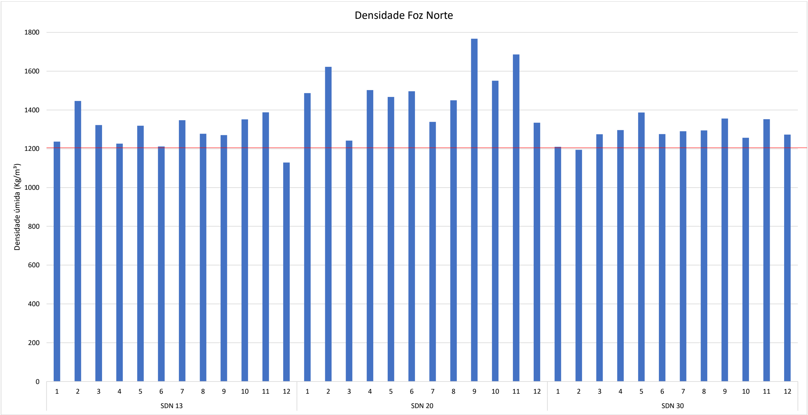
Figura 85: Valores de densidade ( \text{kg/m}^3 ) superficial do Setor Foz Norte. Estações que não apresentaram dados foram decorrentes da ausência de lama no sedimento ou ausência de recuperação de sedimento durante a amostragem.
