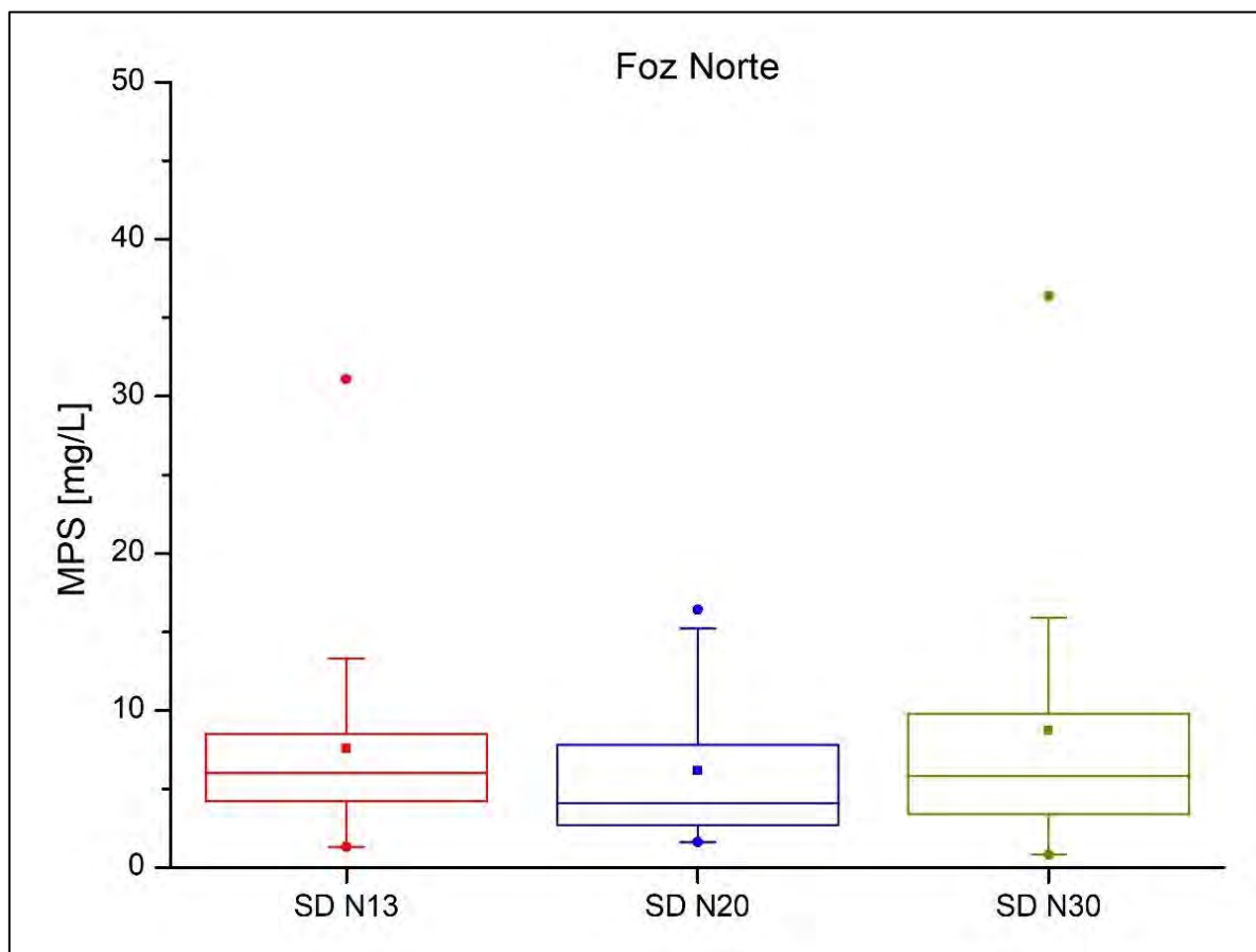
Figura 41: Variabilidade espacial e ao longo da coluna dos valores de MPS para o Setor Foz Norte durante o monitoramento
