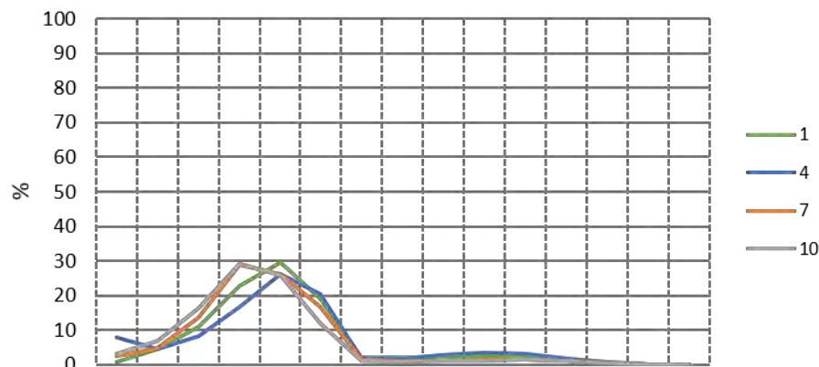
Granulometria CA 03
