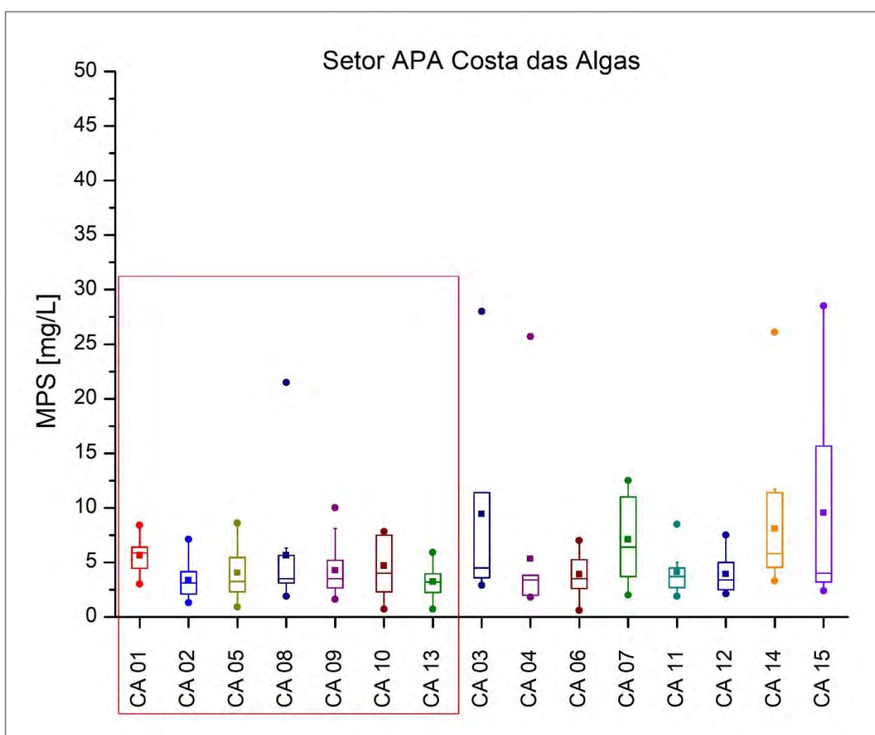
Figura 62: Variabilidade do MPS para as estações do Setor APA Costa das Algas ao longo do monitoramento. Estações rasas se encontram dentro do quadrado vermelho.
