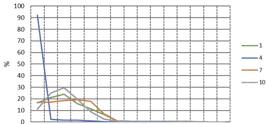
Granulometria CA 12
