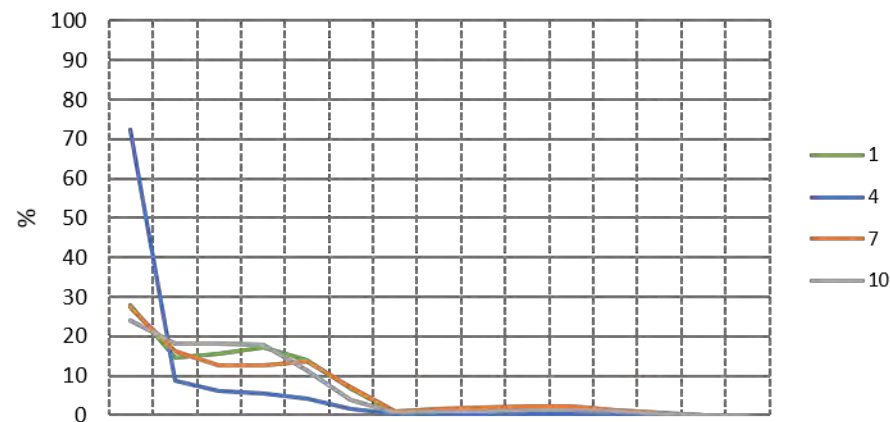
Granulometria CA 15
