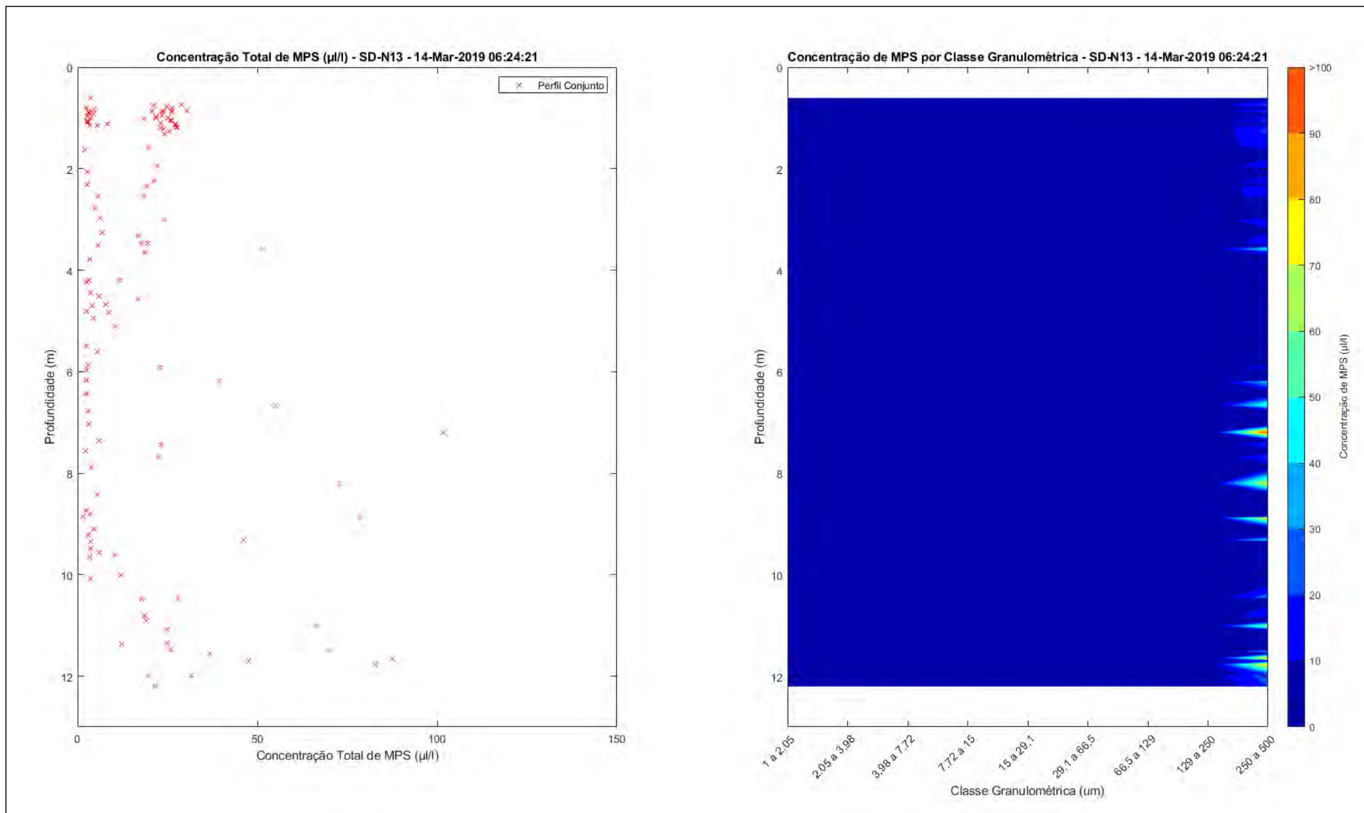
Apêndice 6: Perfisagens realizadas pelo LISST na Campanha 6.
