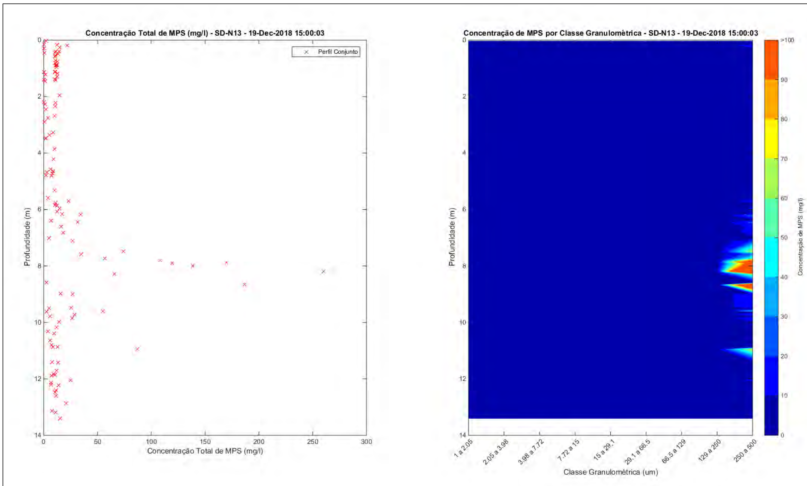
Apêndice 3: Perfisagens realizadas pelo LISST na Campanha 3.
